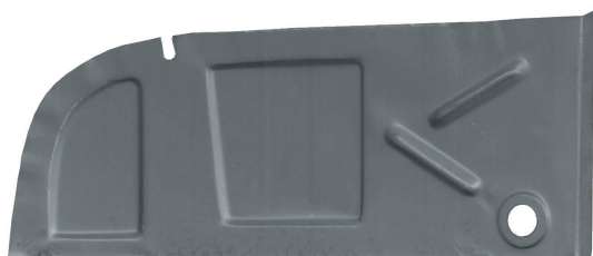
Kieszenie błotników tylnych L/P Inner rear fender repair piece L/R панель пола багажника Л/П
